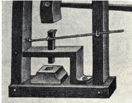
Abb. 2. »Dißes ist der hamer, der uf (die grobe muntz zu muntzen) den stempfel fallen soll, desgleichen das instrument, wie der stempfel eingefast sein soll, mit dem ufheben wider unterzulegen, und wie der underst stempfel in den ambuß gesenckt sein solle.«
