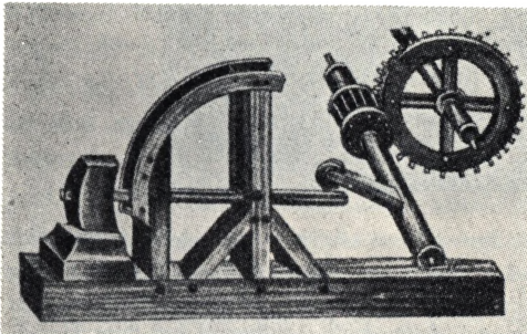
Abb. 3. »Diß ist der wasserhamer, der die plech zu der kleinen sorten der muntz treiben soll, wie hievor auch angeregt.«
