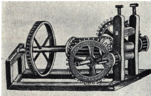
Abb. 6. »Diß ist die ufrichtung der waltzen uf dißem vortzeichneten grund, so er stehen wird, und in ainander gericht, antzusehen ist.« Hier ist also die Verbindung des vorstehenden Wassertriebwerks mit dem kräftigeren Walzwerk dargestellt. Während bei dem Handwalzwerk (Abb. 4) nur die obere Walze gedreht und die untere durch ihren Zahnkranz mitgenommen wird, wird hier jede Walze einzeln angetrieben.
