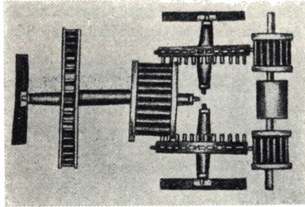
Abb. 5. »Dies ist der grund und antzaigung, das die grossen waltzen treiben soll, ligt im grund, wie es gemacht werden soll, und ain ratgetrieb und drillen in ainander gericht sein sollen.«
