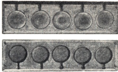
Abb. 1. »Dise ist der model, dorin man die grosse silberne stugk gissen sol. Die Form besteht aus zwei Teilen, die mittelst vier Paßstiften und Löchern zusammengefügt werden. Oben befindet sich eine Gießrinne, von der Eingüsse zu den Einzelformen abgehen.«
